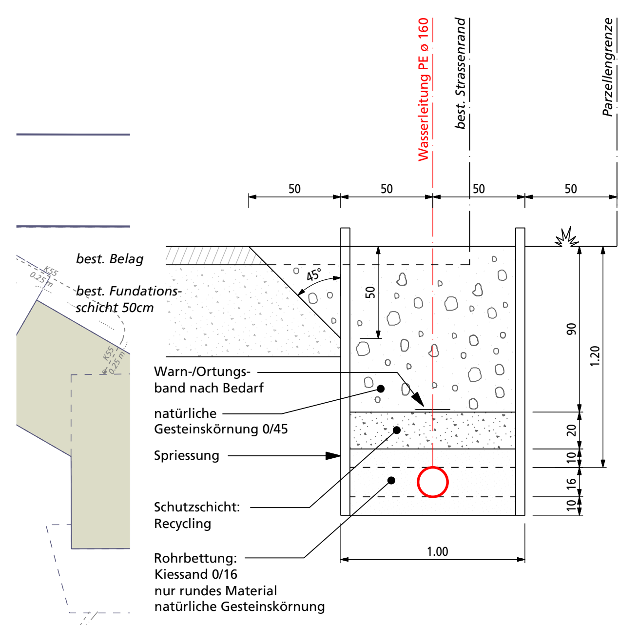
Grabenprofil 1:20 Strasse
