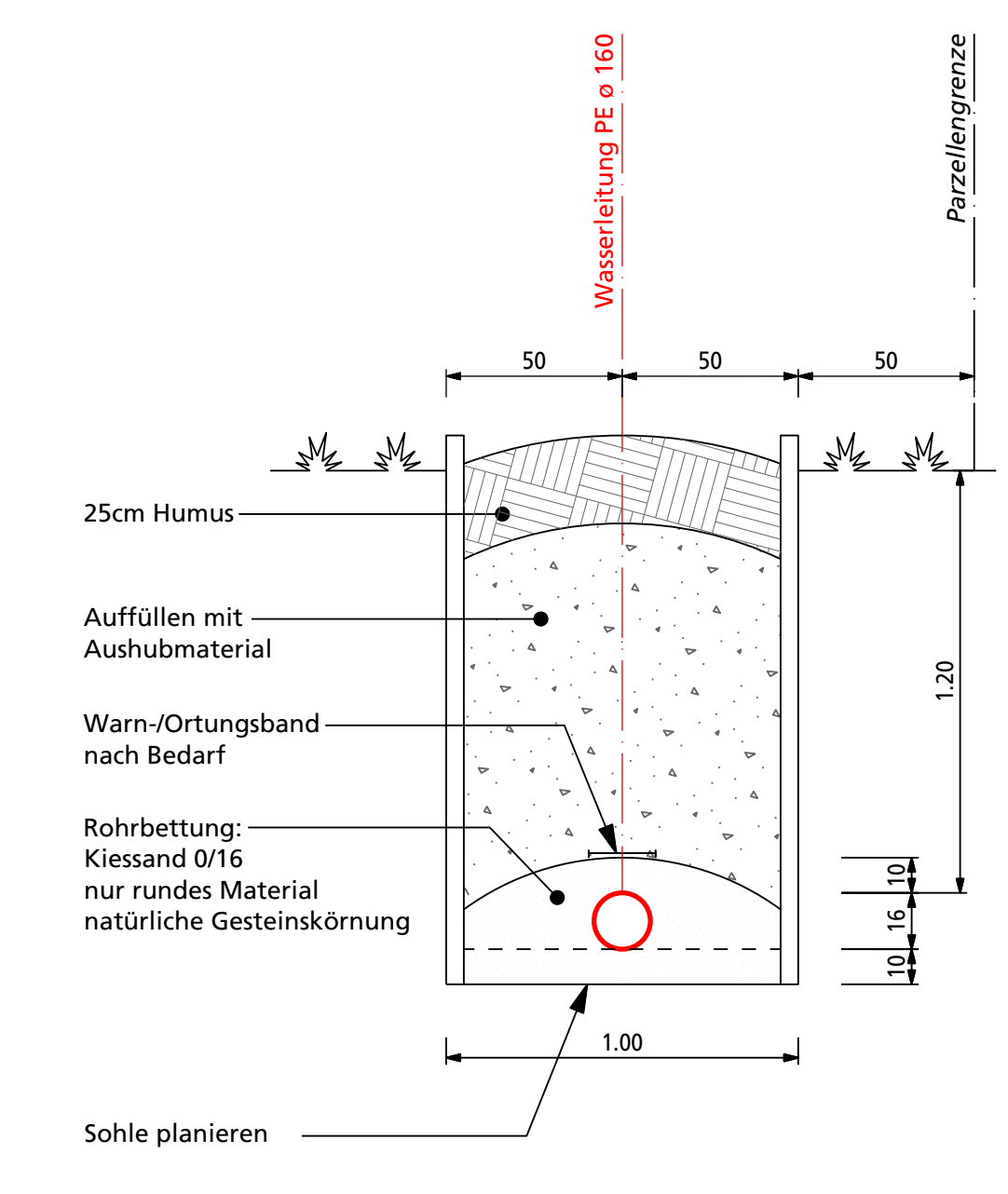
Grabenprofil 1:20 Wiese
