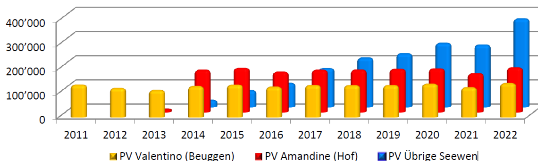
PV Seewen jährlicher Ertrag in kWh
